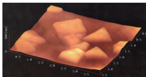
三角形平板状の形態を有する高度好塩性古細菌のAFMイメージ
